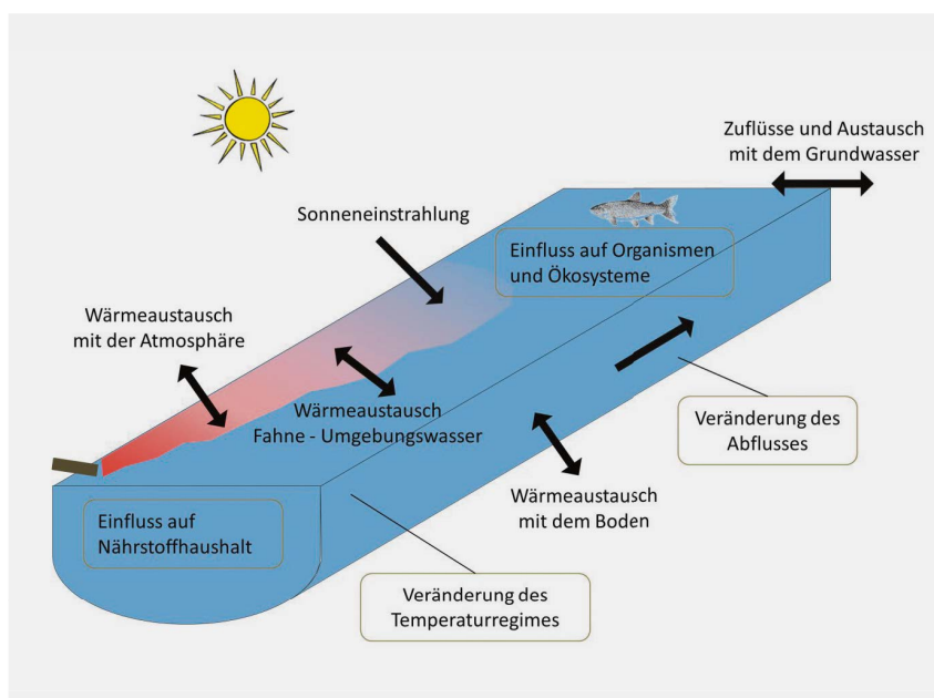
Fig. 2 Thermische Einleitung in ein Fließgewässer: Übersicht über die wichtigsten Wärmeflüsse (Pfeile), die betroffenen Prozesse und möglichen Auswirkungen (eingerahmt).
