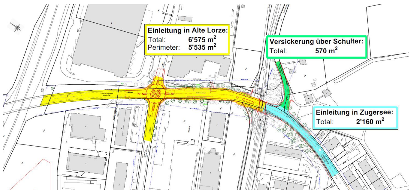
Abbildung 6: Entwässerungssystem
