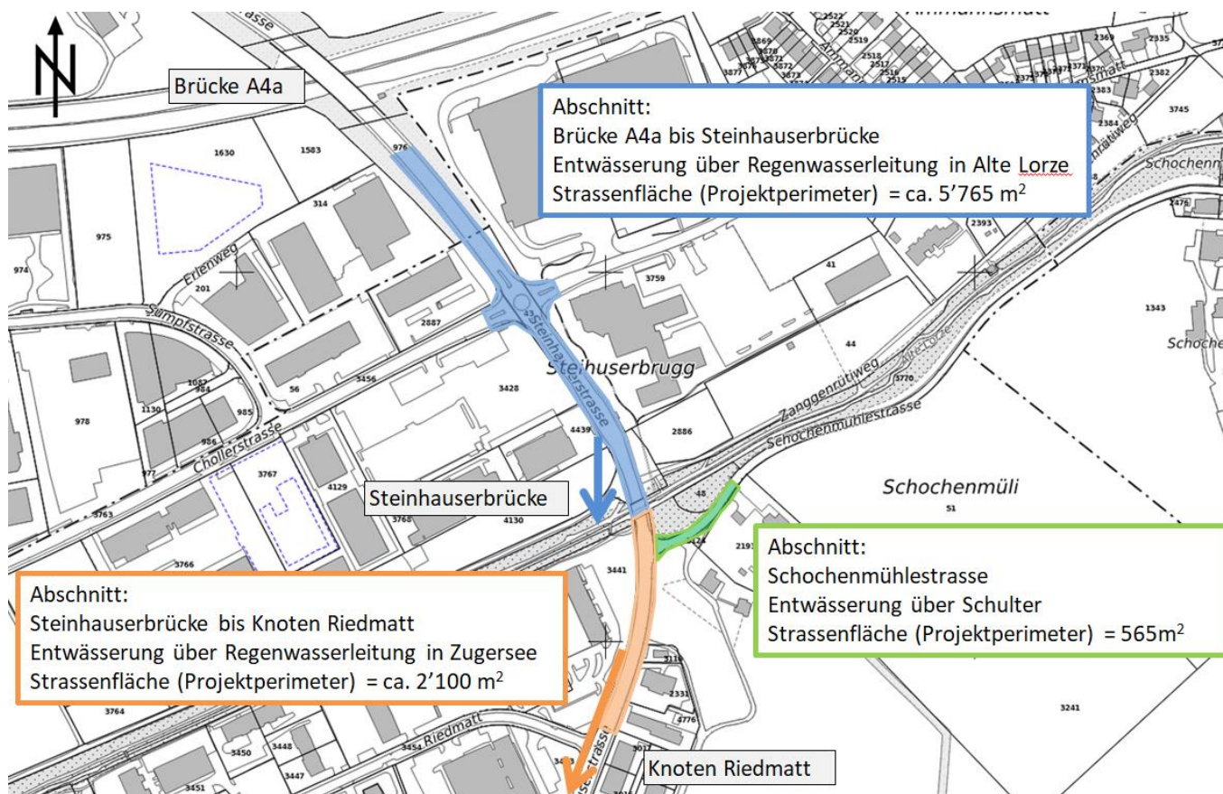
Abbildung 5: Bestehendes Entwässerungsregime
