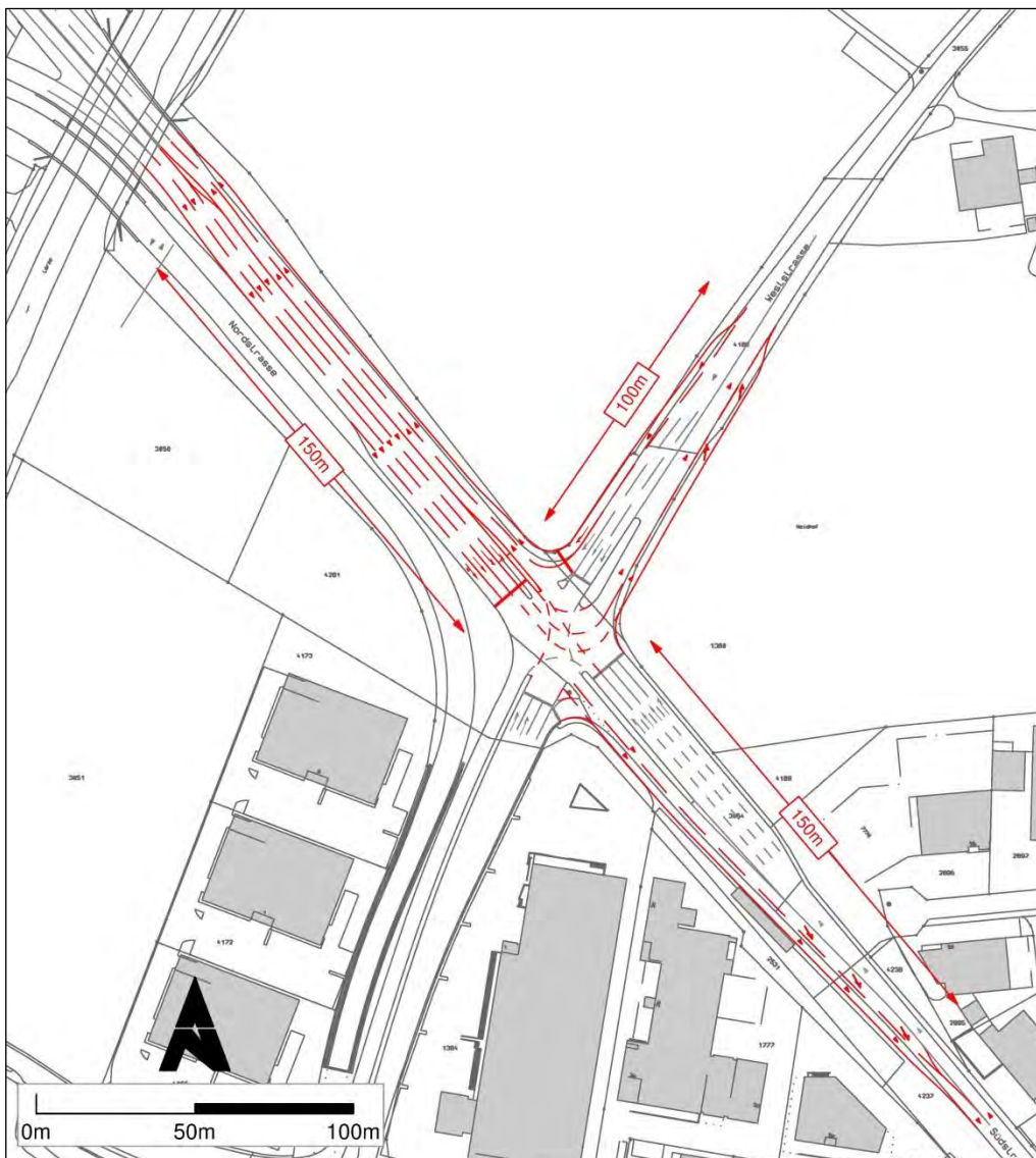
Abbildung 53 Möglicher Ausbau Knoten "Autobahnanschluss" mit niveaugleichem Ausbau
