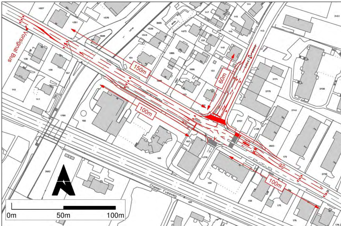
Abbildung 70 Möglicher Ausbau Knoten "Letzistrasse"
