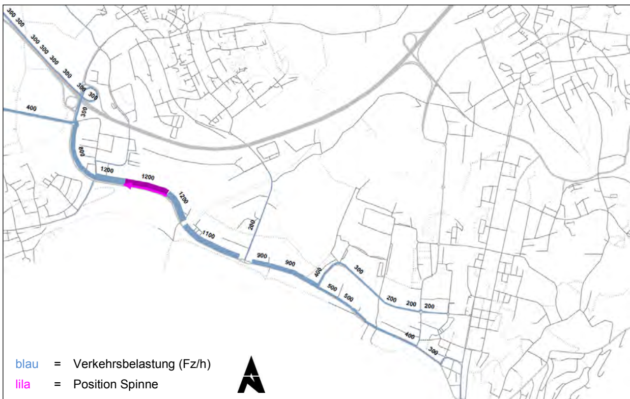
Abbildung 20 Spinne Chamerstrasse, ASP 2030 [ZUG_2015b]
