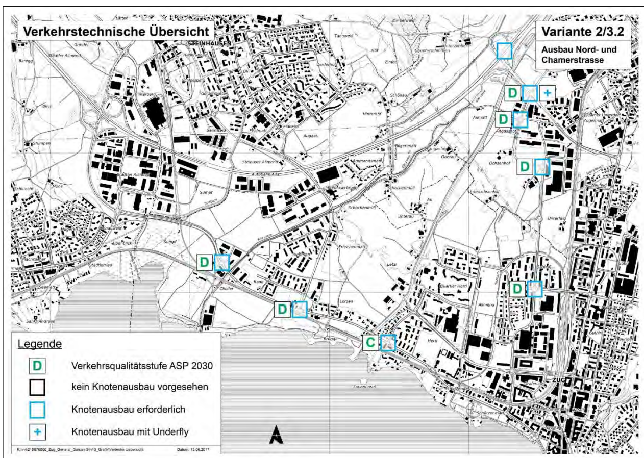
Abbildung 71 Übersicht Variante 2.3
