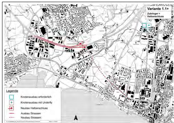
Variante 1.1+: Halbanschluss A4a mit Anbindung an General-Guisan-Strasse
