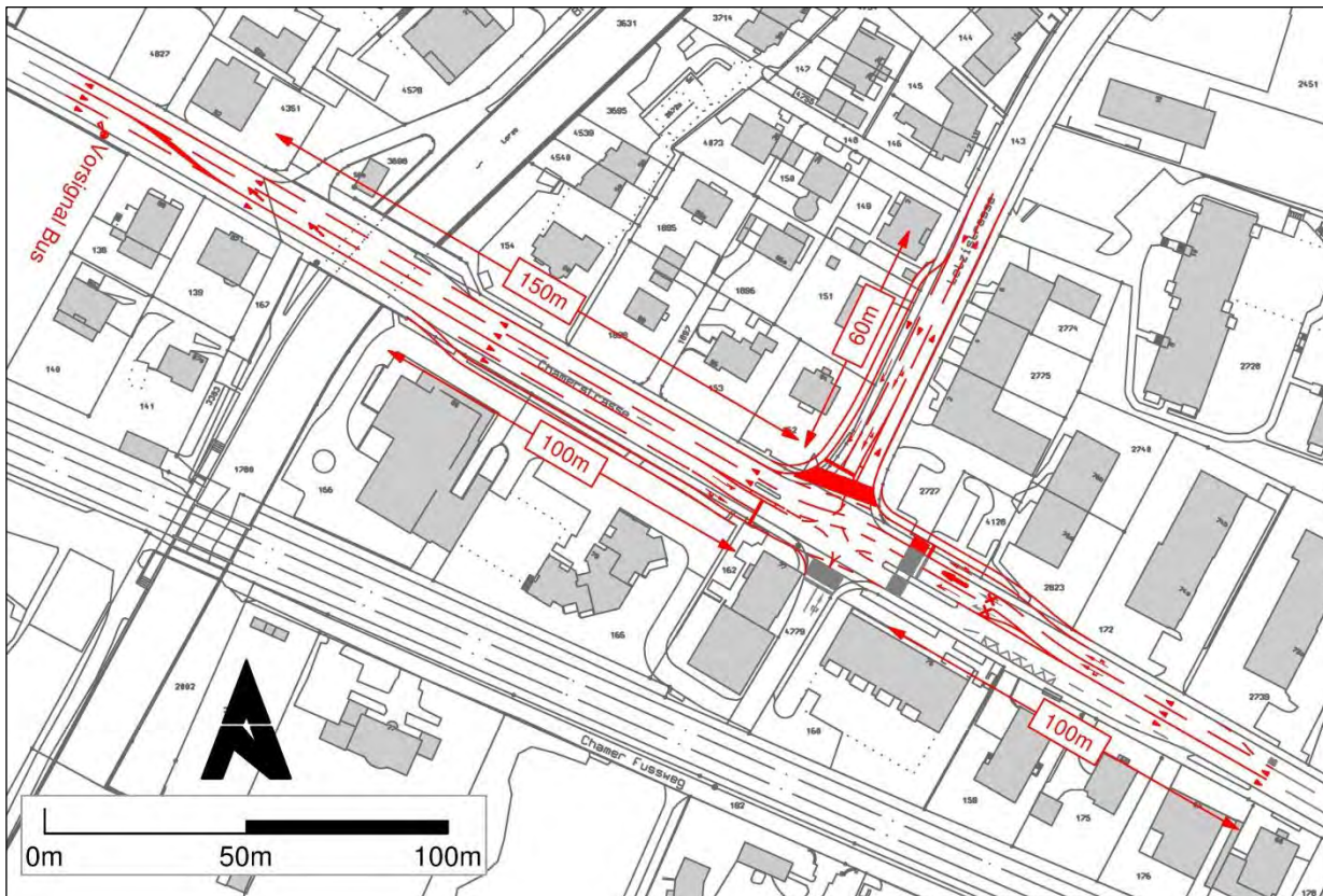
Abbildung 56 Möglicher Ausbau Knoten "Letzistrasse"
