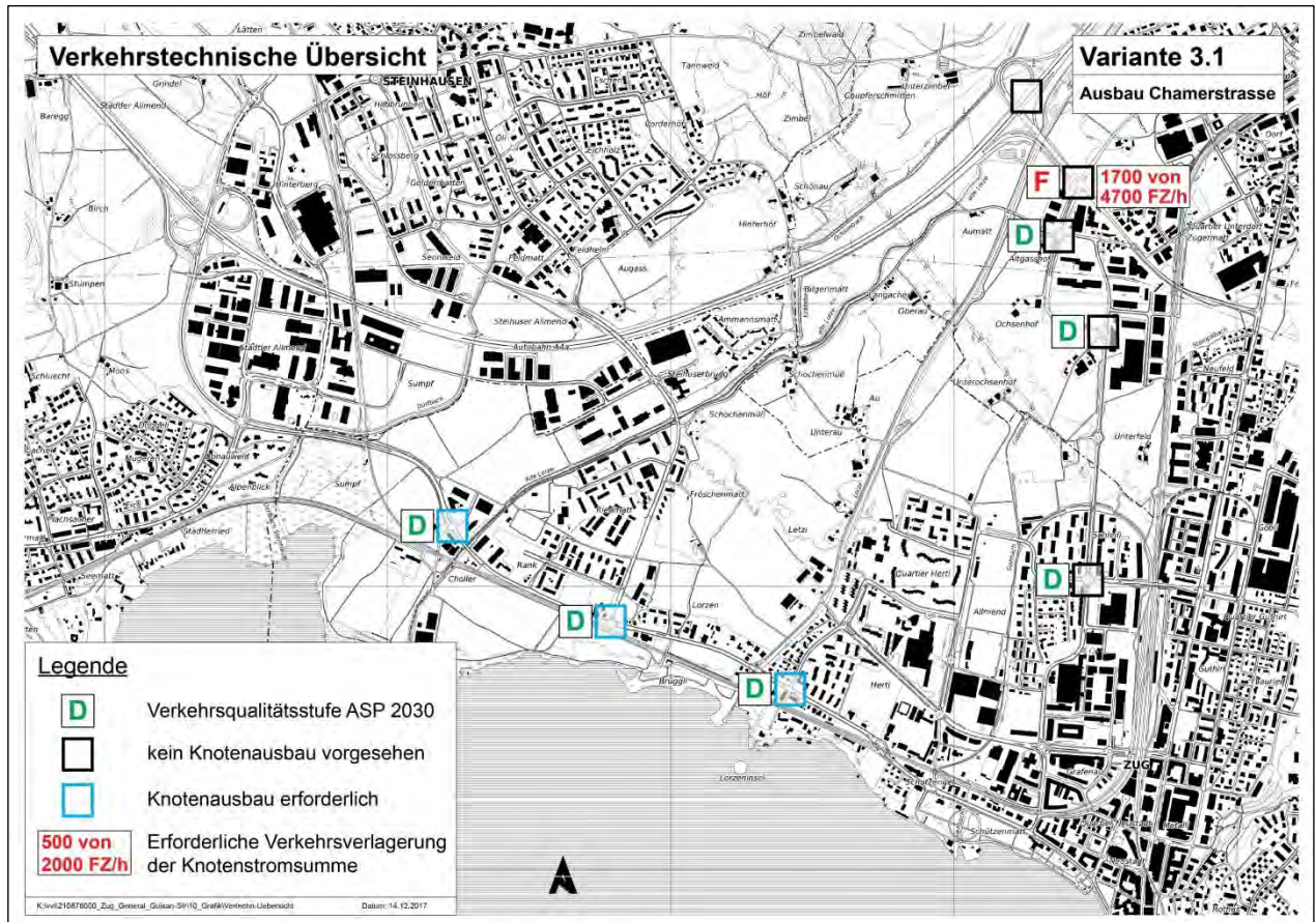
Abbildung 67 Übersicht Variante 3.1
