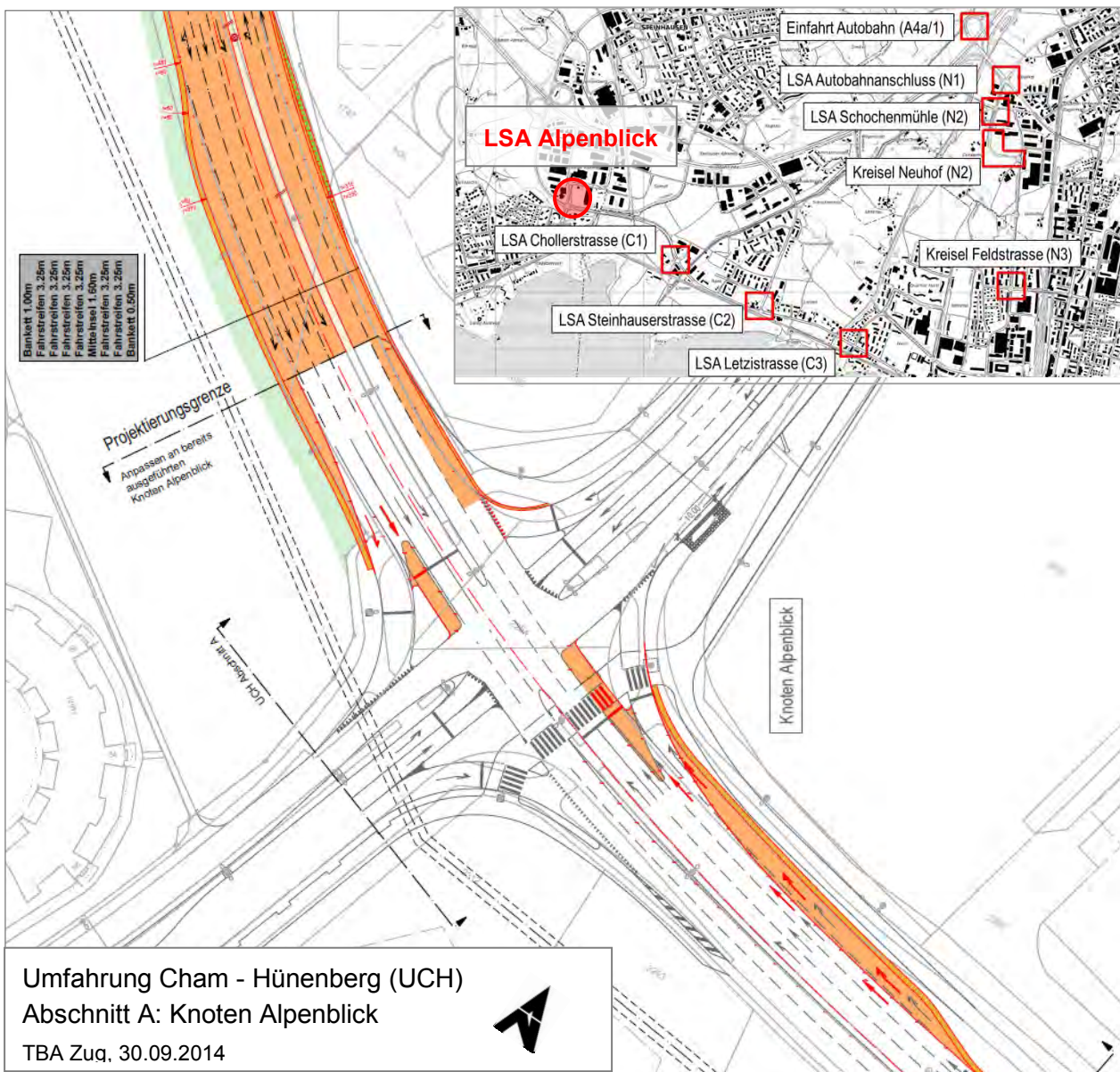
Abbildung 14 LSA Knoten Alpenblick gemäss Auflageprojekt UCH
