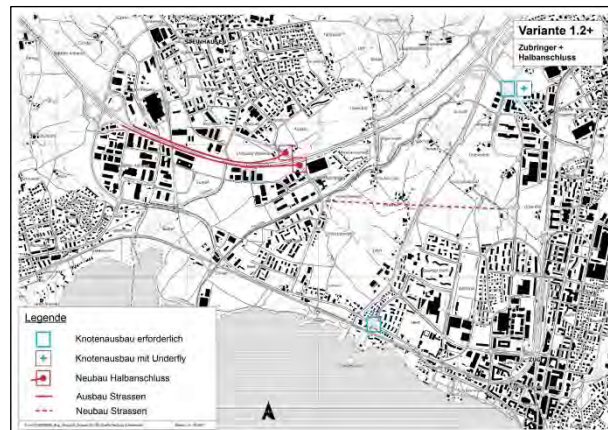
Variante 1.2+: Halbanschluss A4a mit Anbindung an die Nordstrasse
