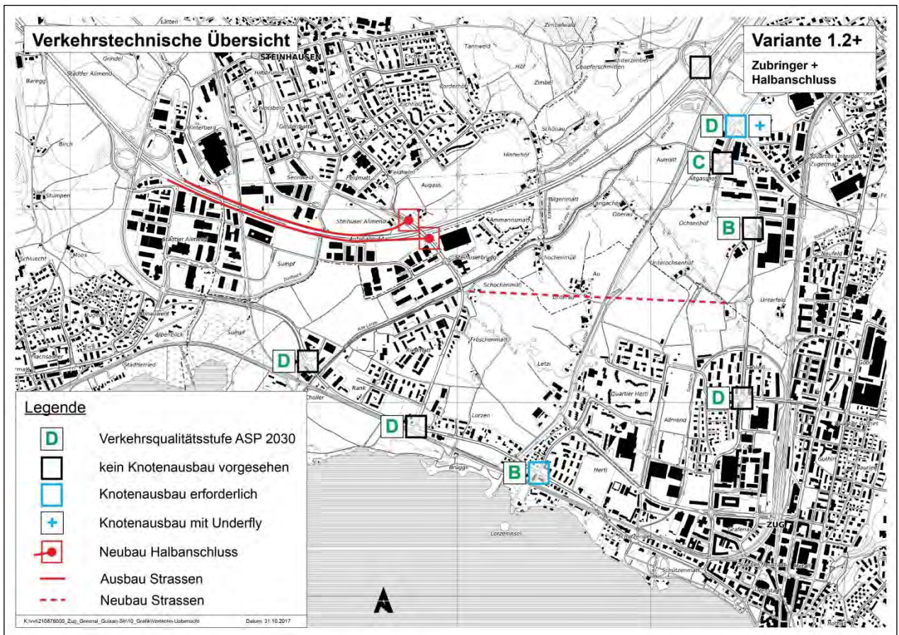
Abbildung 57 Verkehrstechnische Übersicht Variante 1.2+ (ASP 2030)
