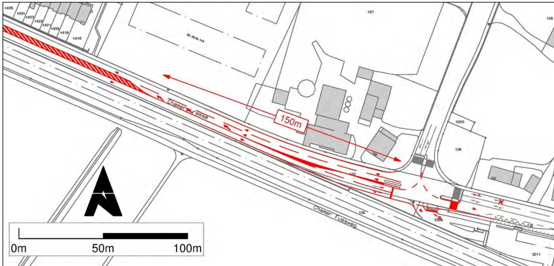
Abbildung 69 Möglicher Ausbau Knoten "Steinhauserstrasse"
