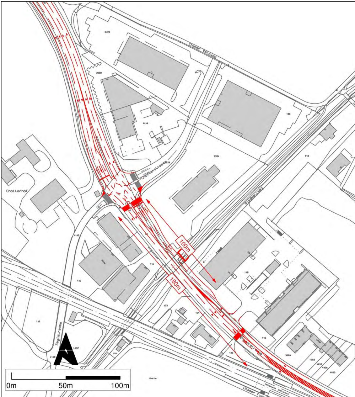
Abbildung 68 Möglicher Ausbau Knoten "Chollerstrasse"
