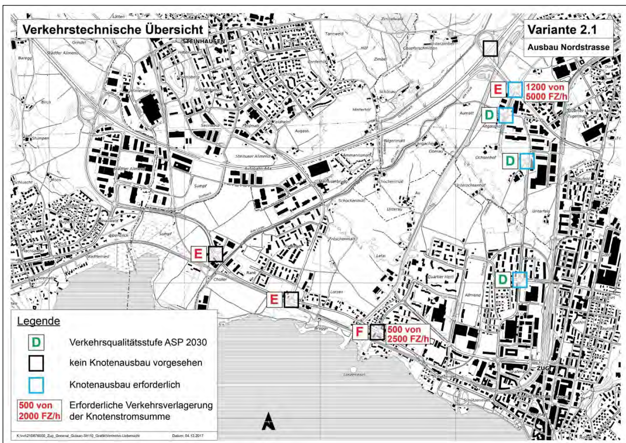
Abbildung 62 Übersicht Variante 2.1
